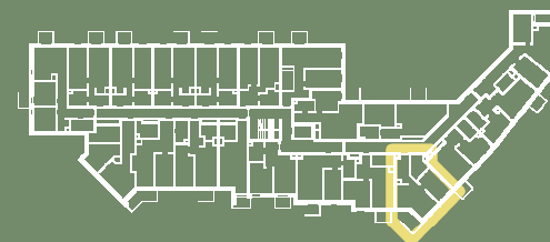
SCHEMAT KONDYGNACJI
